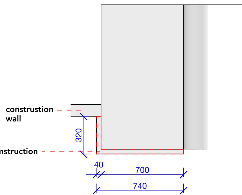
section B-B' M 1:20
